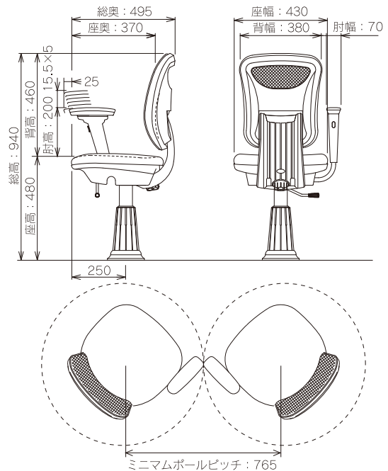
MD-2630(W) フルアジャスタブル (可動) アームレスト (オプション) 仕様
