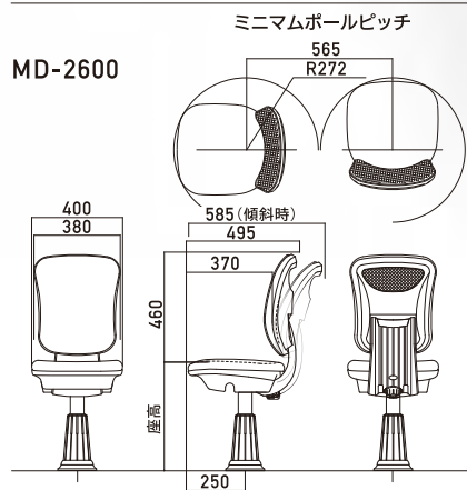
寸法図 (mm) ※寸法は理論値のため±10mm程度の誤差が生じます。
